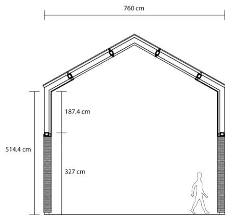
影像穿廊剖面圖
